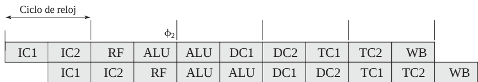
(a) Implementación supersegmentada del cauce optimizado del R3000
