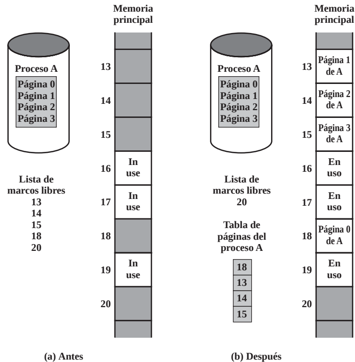
Figura 8.15. Asignación de marcos libres.
