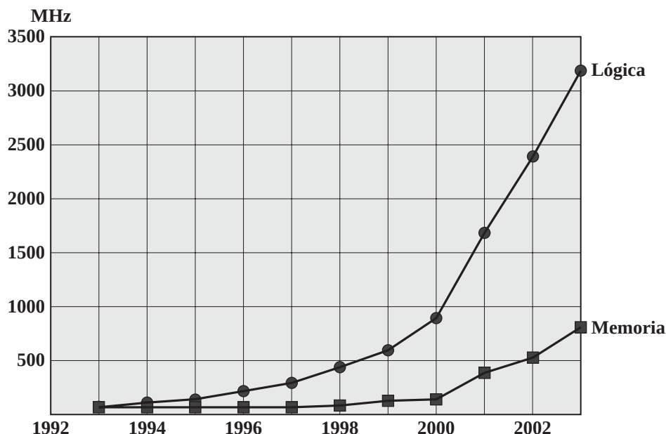
Figura 2.10. Prestaciones de la memoria y la lógica [BORK03].
