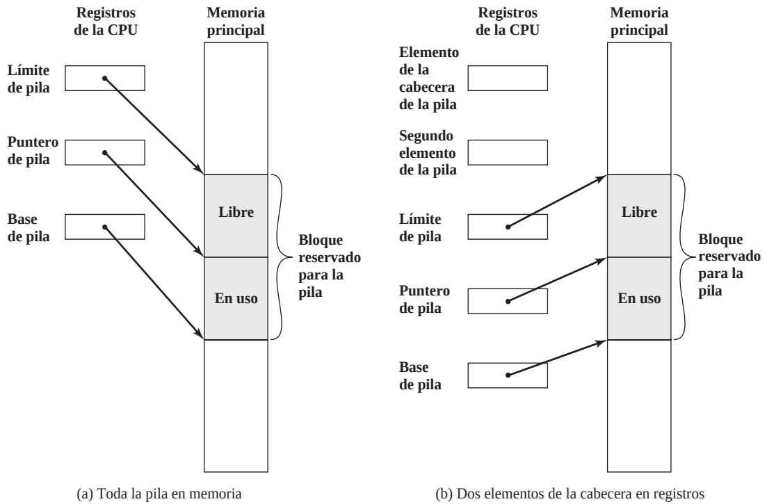
Figura 10.14. Organizaciones de pila usuales.
