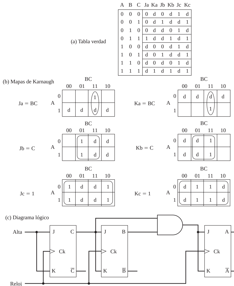
Figura B.33. Diseño de un contador síncrono.
