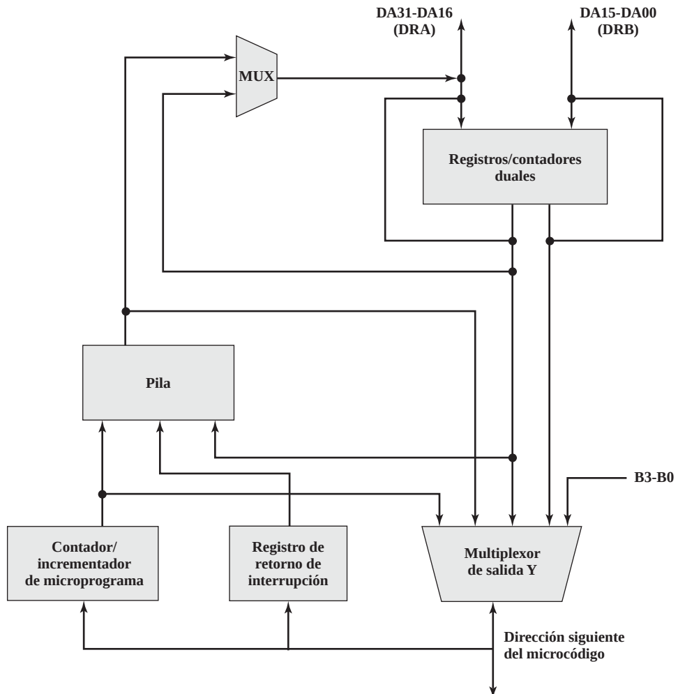
Figura 17.18. El microsecuenciador TI 8818.
