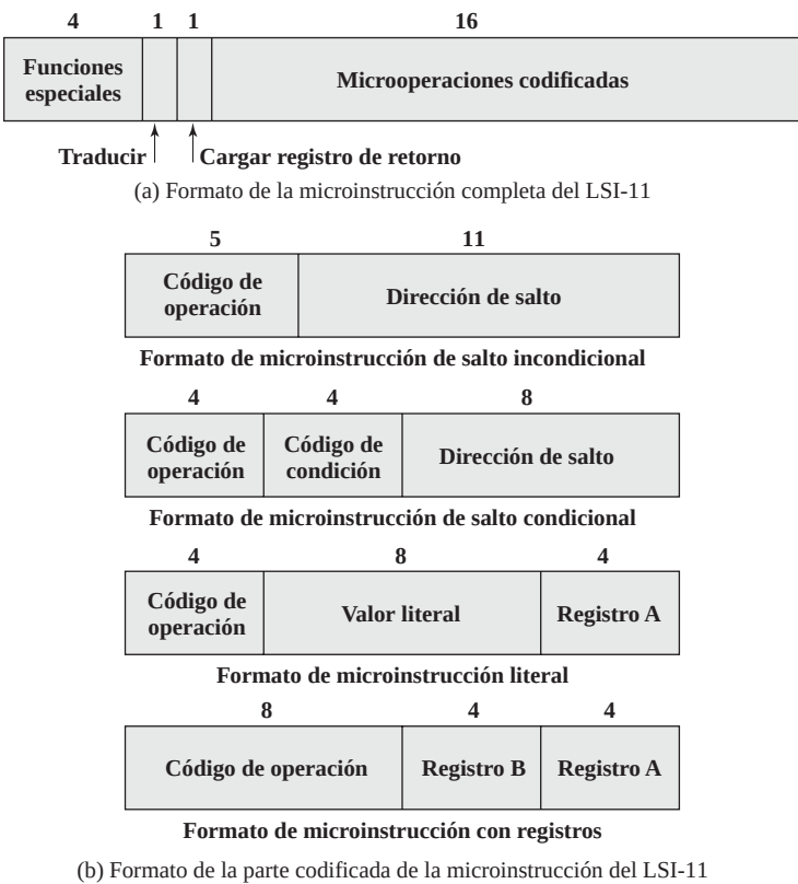
Figura 17.15. Formato de microinstrucción del LSI-11.
