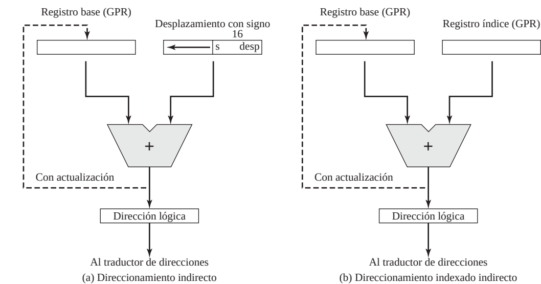
Figura 11.3. Modos de direccionamiento de operandos en memoria del PowerPC.
