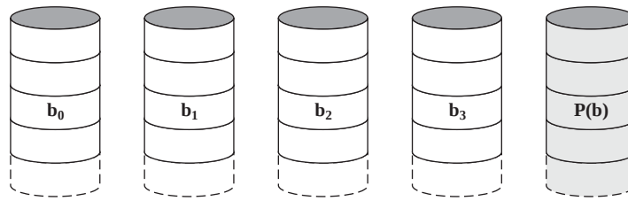
(a) RAID 3 (bit de paridad intercalada)
