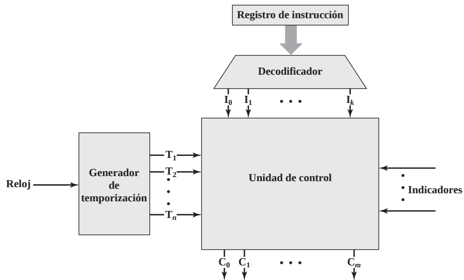
Figura 16.10. Unidad de control con entradas decodificadas.
