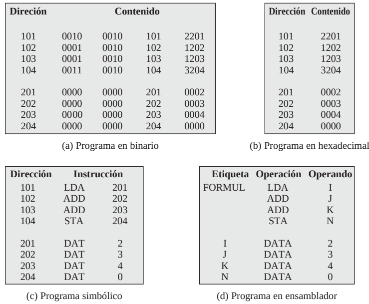
Figura 10.11. Cálculo de la fórmula N = I + J + K .
