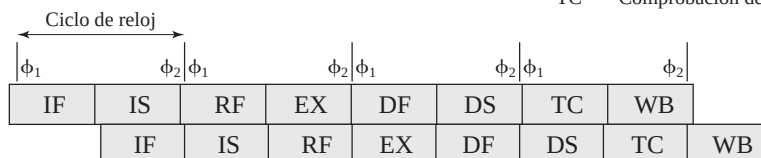
(b) Cauce del R4000
