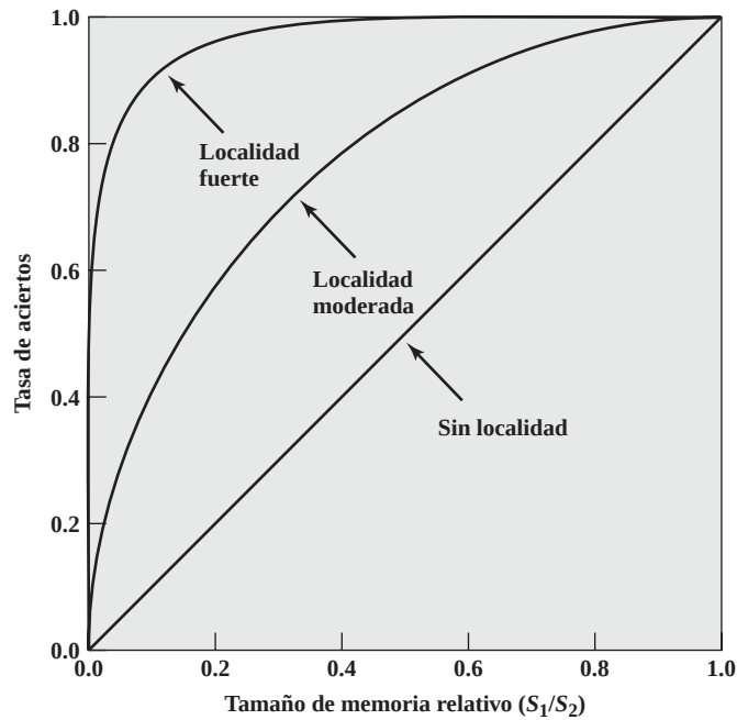
Figura 4.20. Tasa de aciertos en función del tamaño relativo de las memorias.
